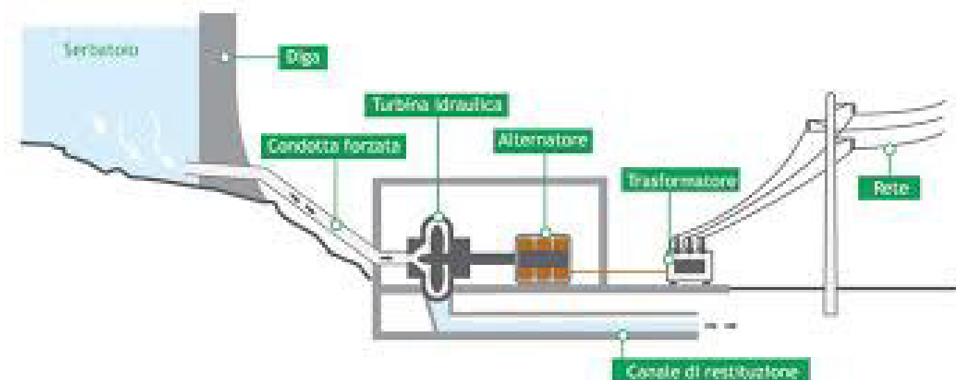
Nella Figura: impianto idroelettrico
