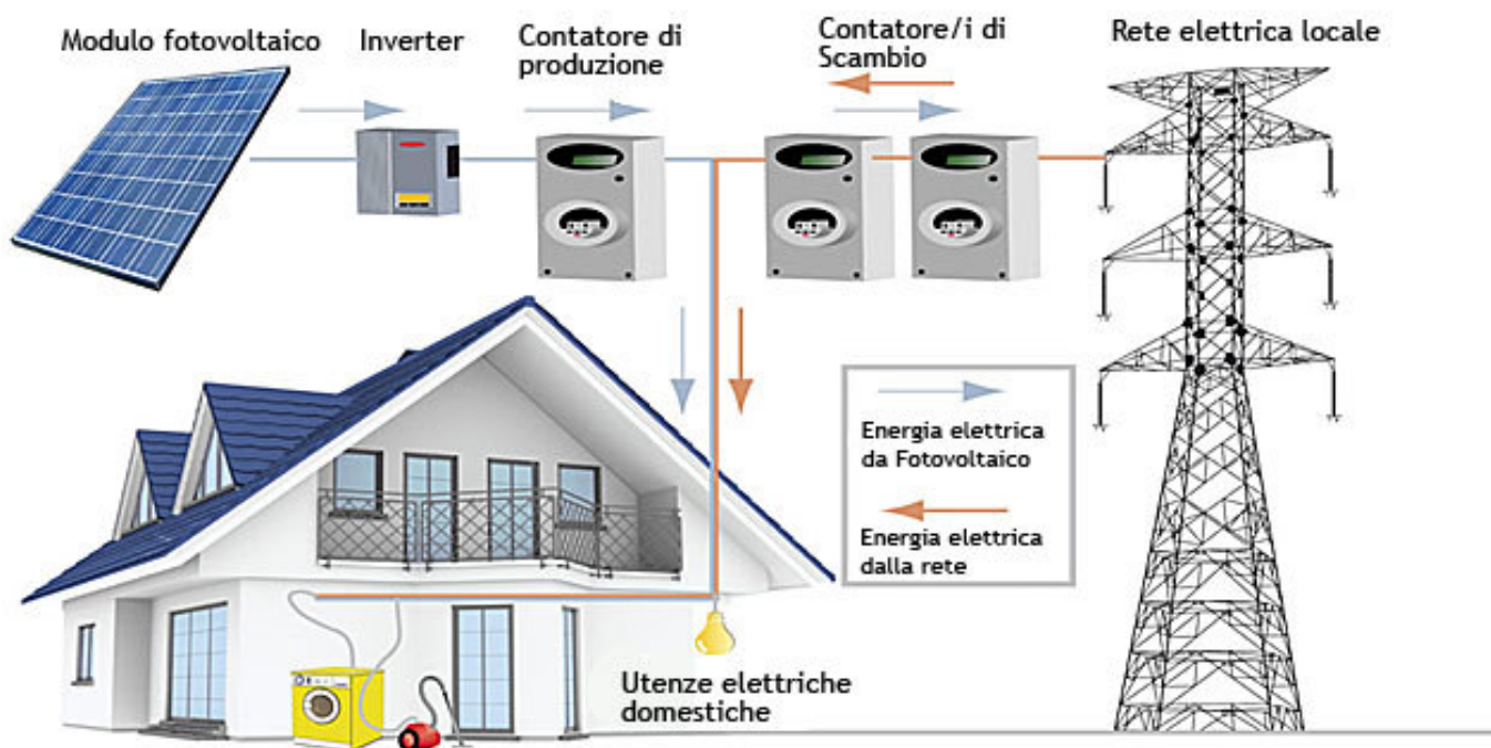
Nella Figura: impianto solare fotovoltaico
